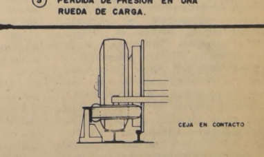
EL METRO sobre neumáticos tiene, como elemento básico de rodamiento, una carretilla (bogie o truck) de características especiales. Esto permite eliminar notablemente las vibraciones, lo que significa un alto grado de comodidad para el público y mayor durabilidad de los vehículos en comparación con los sistemas convencionales. El rodado de goma permite, además, hacer más expedito el frenado. Su seguridad está respaldada por ruedas provistas de mallas de acero. La foto superior y los dibujos muestran el perfecto del sistema.
