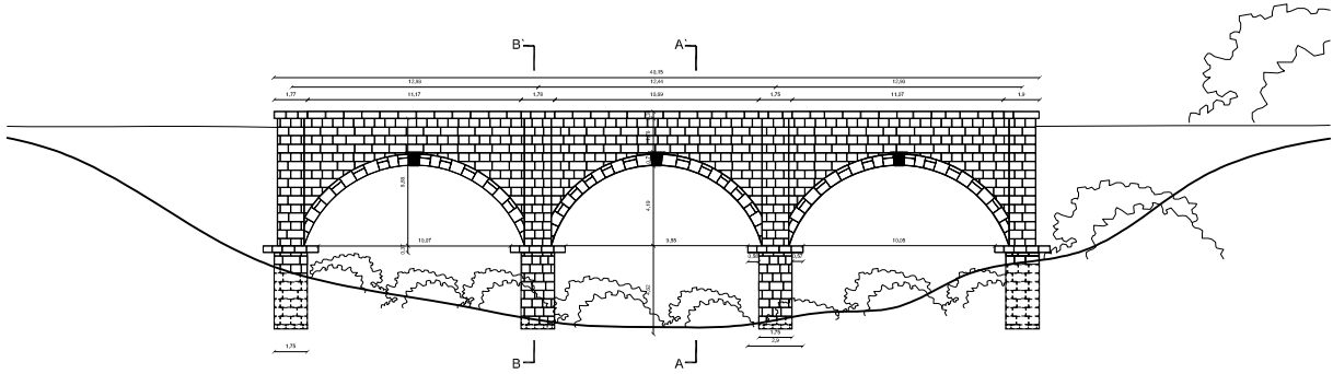
ELEVACIÓN PONIENTE Escala Gráfica
