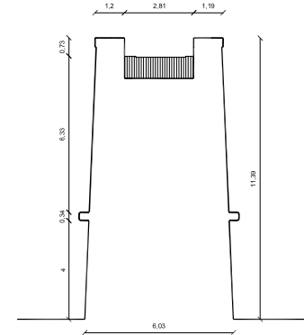
CORTE B - B' Escala Gráfica
