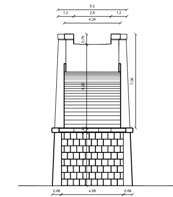
CORTE A - A' Escala Gráfica
