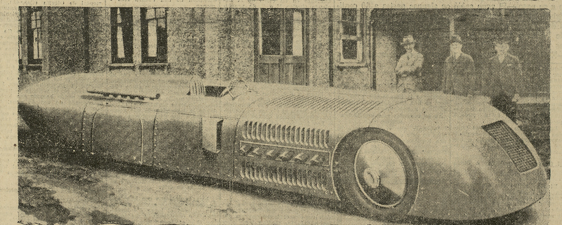
Con esta formidable máquina, accionada por dos motores de 500 caballos, el piloto inglés mayor Segrave, proyecta batir todos los records americanos en una pista de EE. UU. Cree que podrá alcanzar la velocidad de 400 kilómetros por hora
