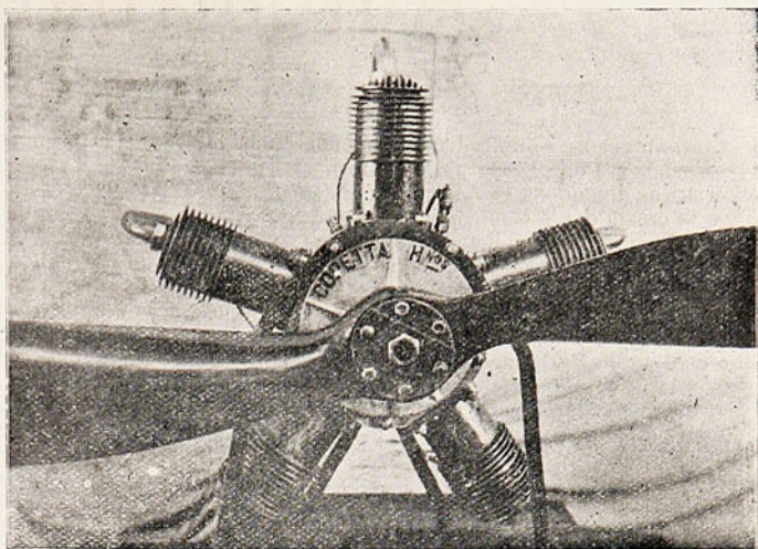
El motor visto de frente
