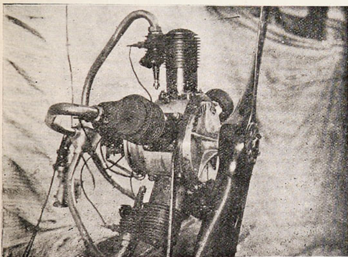
El motor visto de costado
