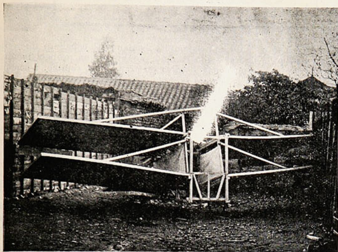
Vista general del modelo de biplano
