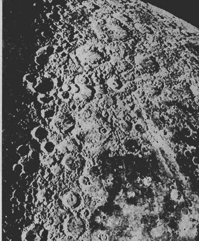
"Las tierras malas de la Luna". — Parte sur del planeta en cuarto menguante (Reproducción fotográfica del Observatorio de M. Wilson)
