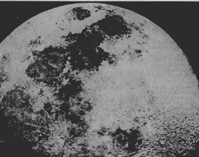
La Luna, pasado el primer cuarto (reproducción fotográfica del Observatorio Lick)
