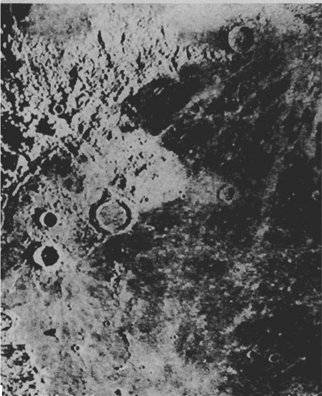
"Mar de las lluvias". — La Luna en cuarto menguante (Reproducción del Observatorio de M. Wilson)
