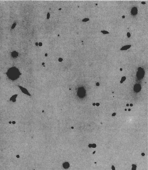
Un grupo de galaxias, situadas a 500 millones de años-luz, fotografiadas en el Observatorio de Monte Palomar
