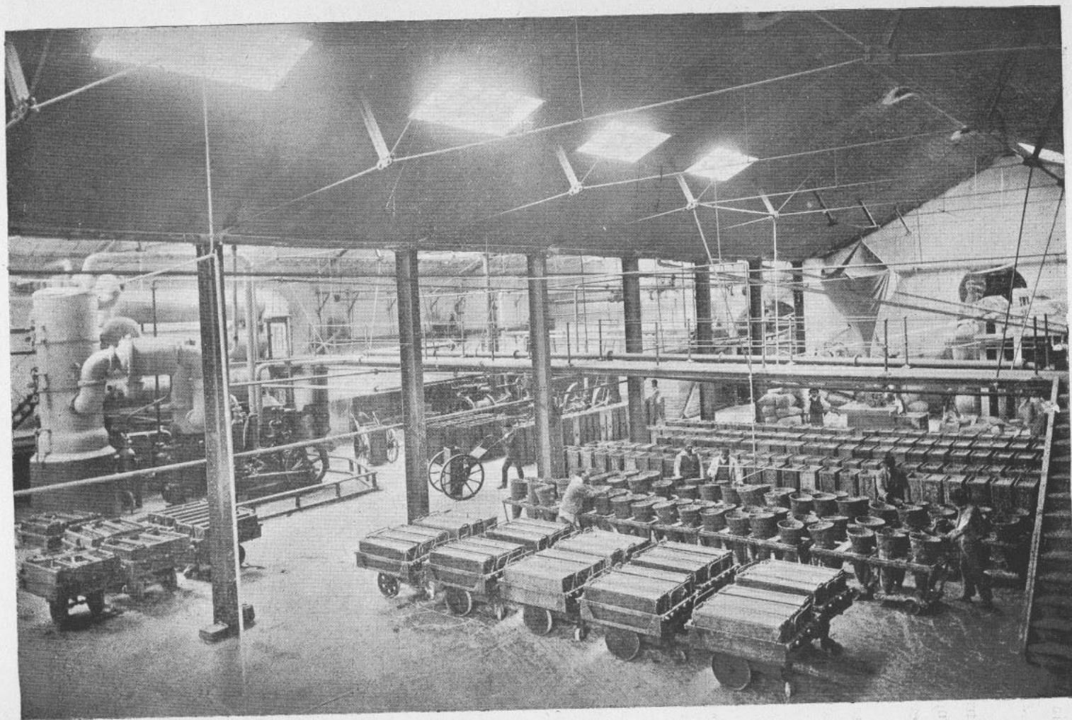
REFINERÍA DE AZÚCAR — VIÑA DEL MAR. — SECCIÓN «TRIPLE EFECTO» Y «MOLDES»
