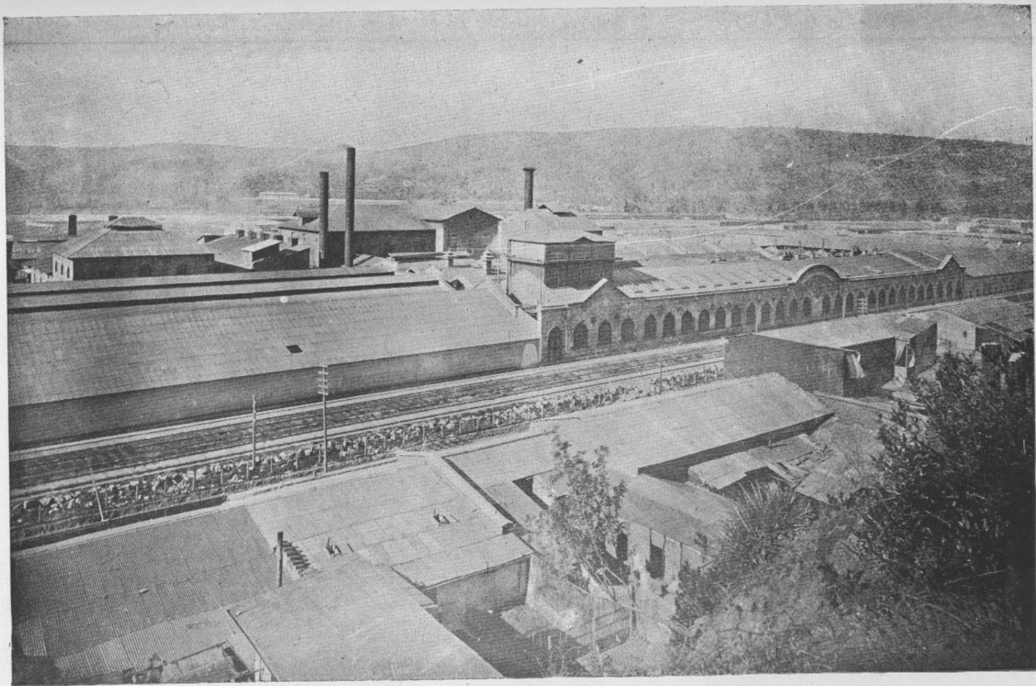
REFINERÍA DE AZÚCAR — VIÑA DEL MAR — VISTA EXTERIOR
