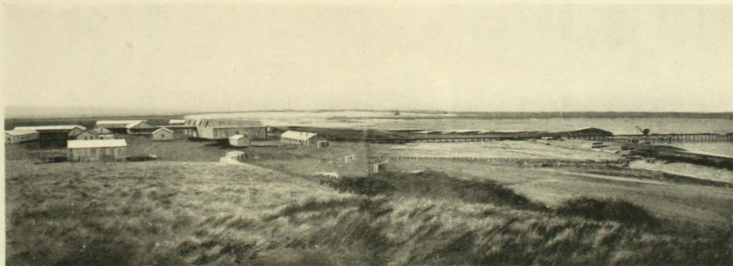
Panorama de las instalaciones de la «Compañía Frigorífica de Patagonia. Puerto Sara. Bahia San Gregorio
