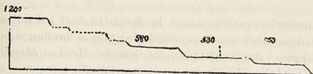
Fig. 2.—Corte de los llanos en la bahía San Jorje.
