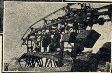
Una filovia per il trasporto del zolfo greggio dal monte Chupiquiña (m. 5.800)
