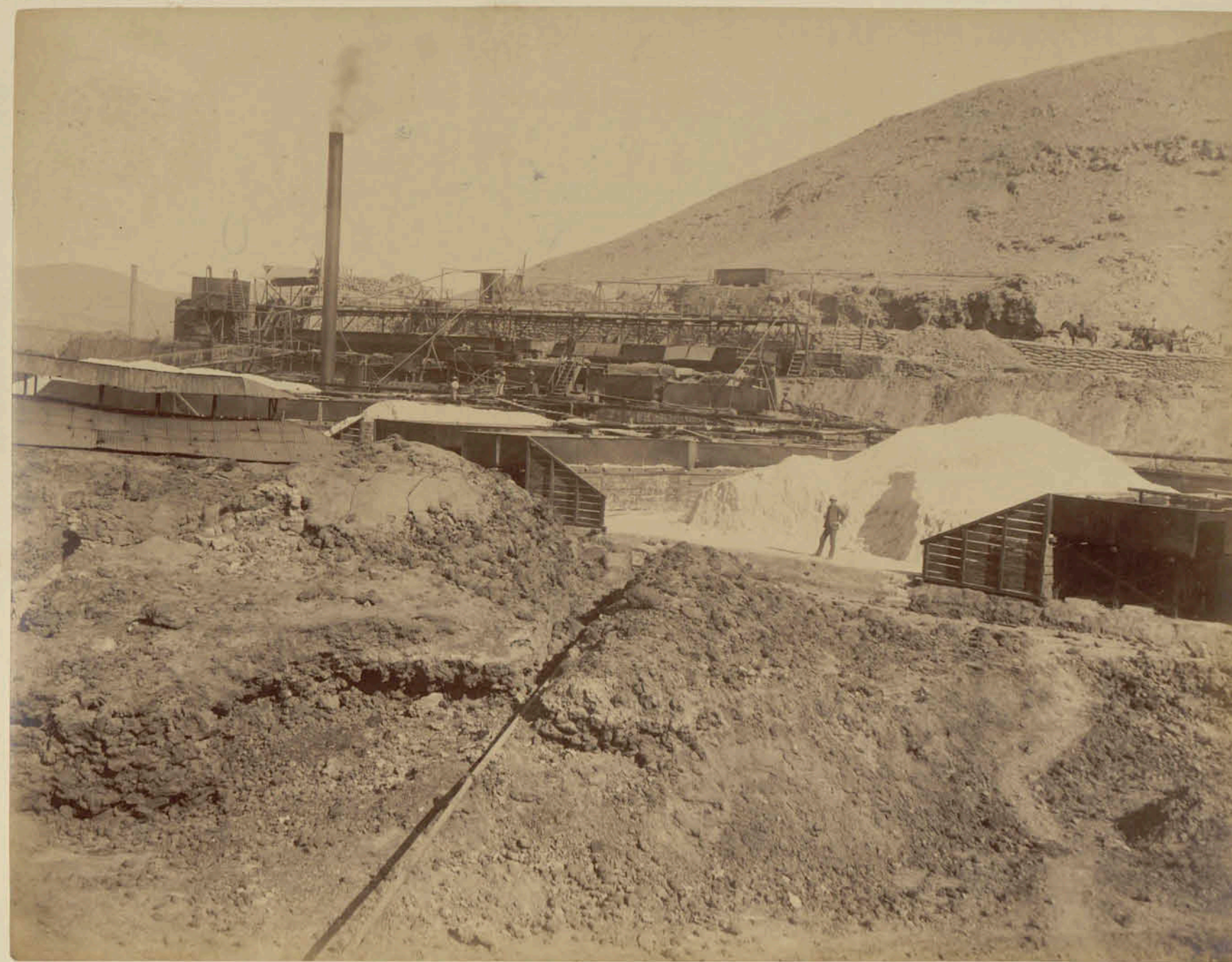
Oficina Aurora MAQUINARIA
